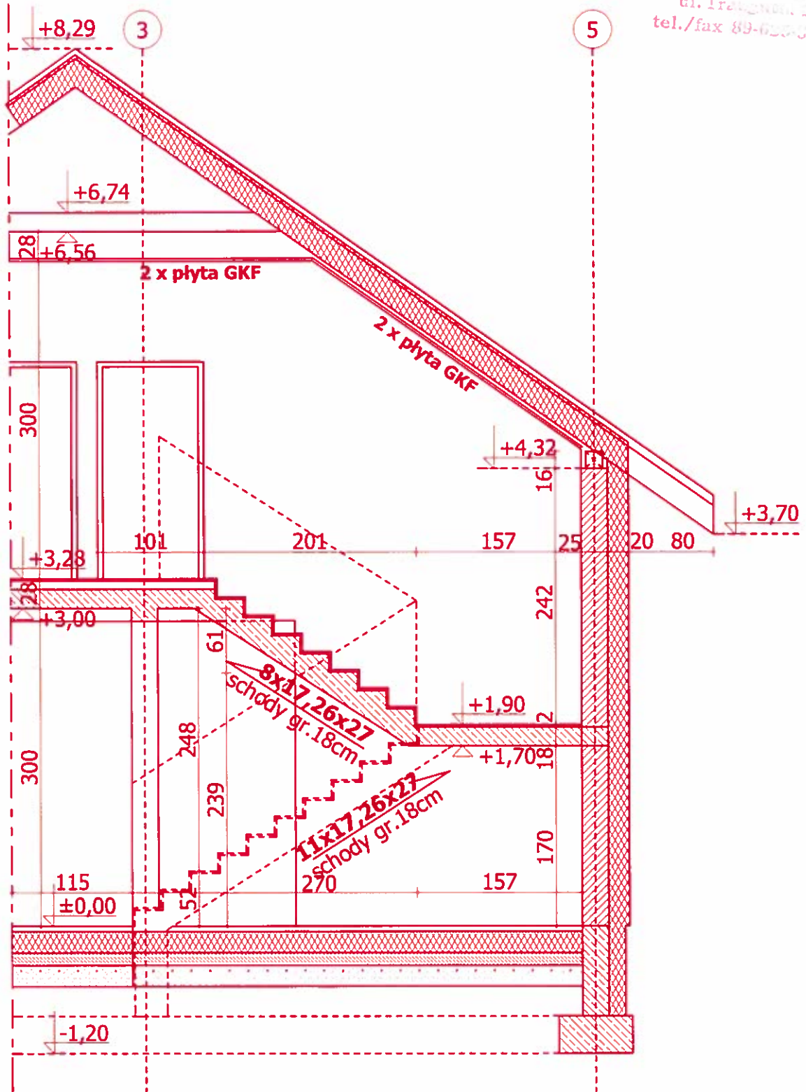
PRZEKRÓJ PRZEZ SCHODY skala 1:50
